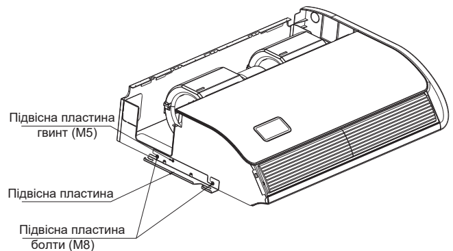
мал. 3.3.6 Болти підвісу
