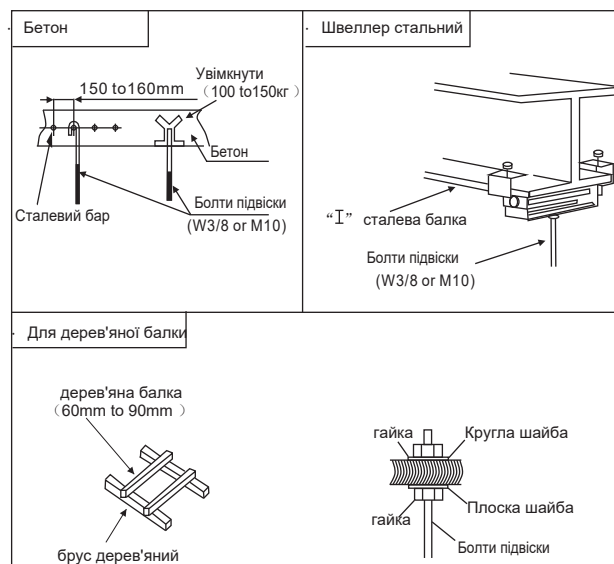
Мал. 3.3.1 Кріплення болтів підвіски
